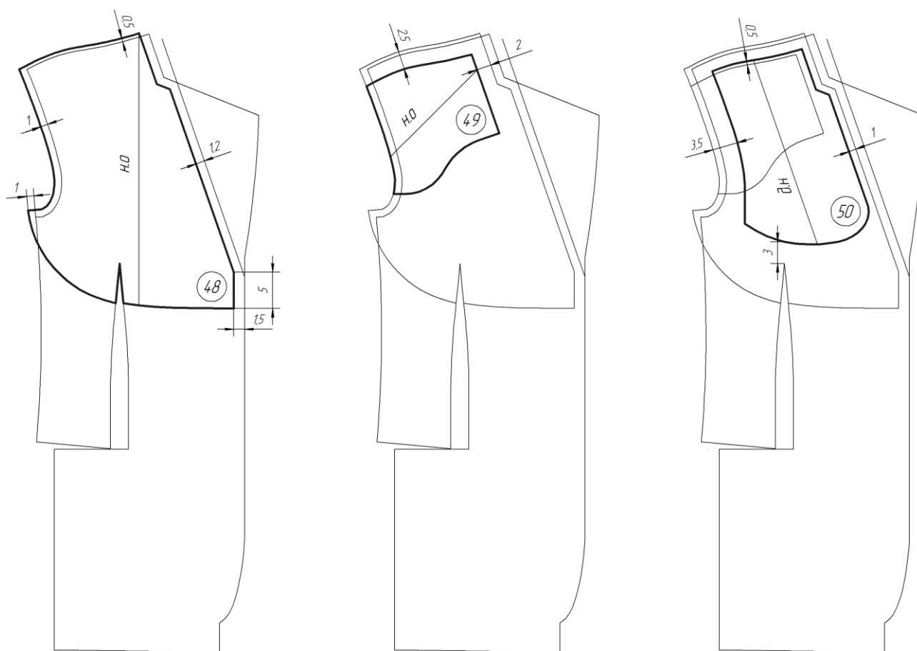
Рисунок 14. Производные лекала из прокладочной ткани мужского пиджака
